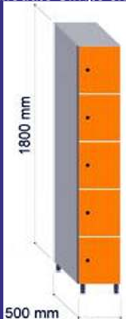
ANCHO 200-250-300-400-500
